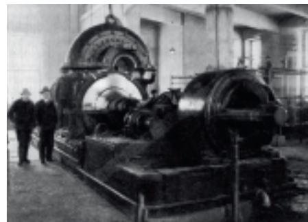
Montaż polskiego alternatora z publikacji 400 lat Poczty Polskiej
